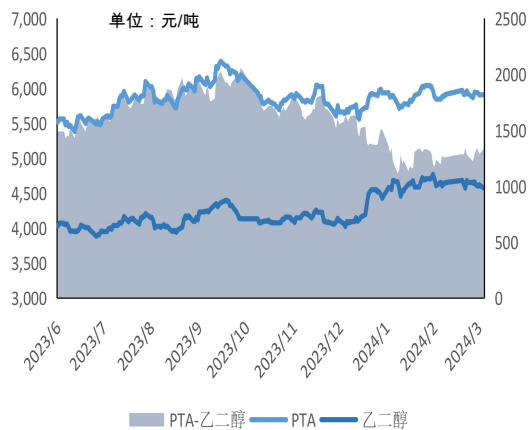
图5：PTA-MEG价差
