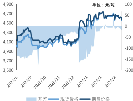
图2：期现价差
